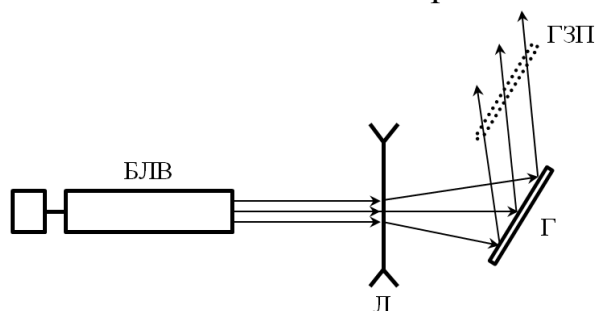
Рис. 5. Схема установки для відтворення голограм: БЛВ – блок лазерного випромінювання (лазер і блок живлення); Л – розсіювальна лінза; Г – голограма; ГЗП – голографічне зображення предмета.
