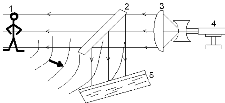
Рис. 1. Найпростіша схема запису голограми: 1 – об’єкт; 2 – напівпрозоре дзеркало; 3 – розширювач променя; 4 – лазер; 5 – світлочутлива пластинка.
