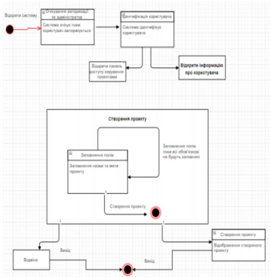
Рисунок 2.3 – Діаграма станів для створення проекту
