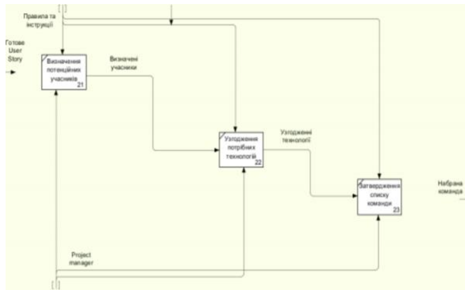
Рис. 1.3 – Діаграма процесу створення команди
