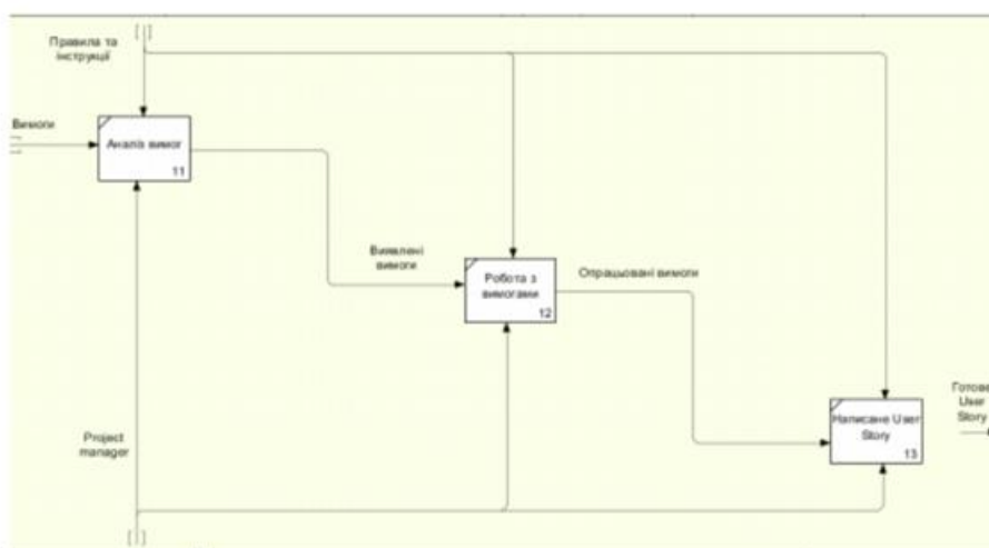
Рис. 1.1 – Діаграма бізнес-процесів розроблюваного програмного продукту.
