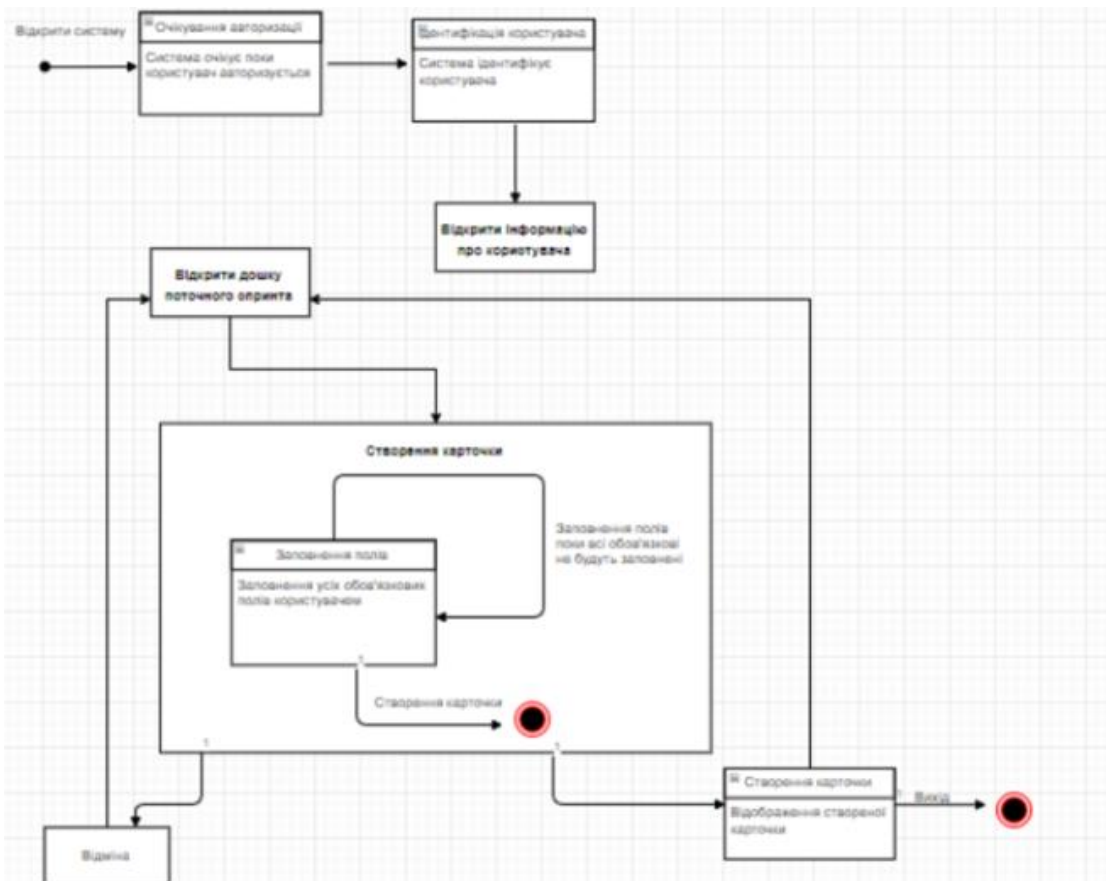
Рис. 2.5 – Діаграма станів для створення картки
