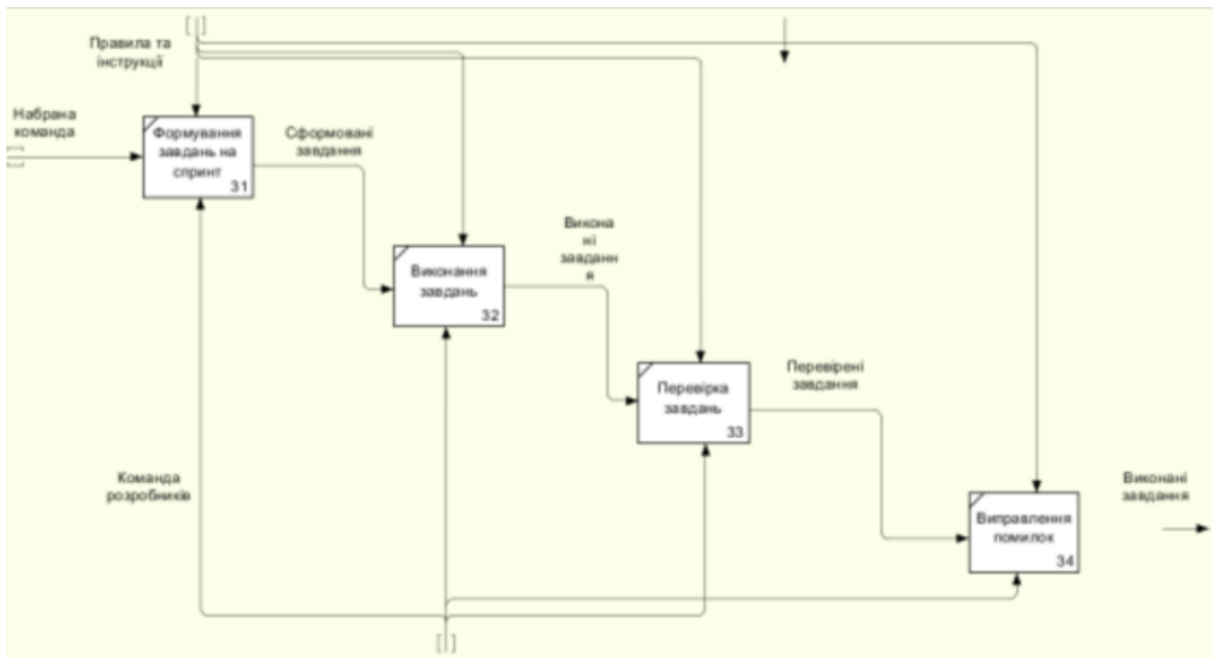
Рис. 1.4 – Діаграма процесу роботи зі спринтом
