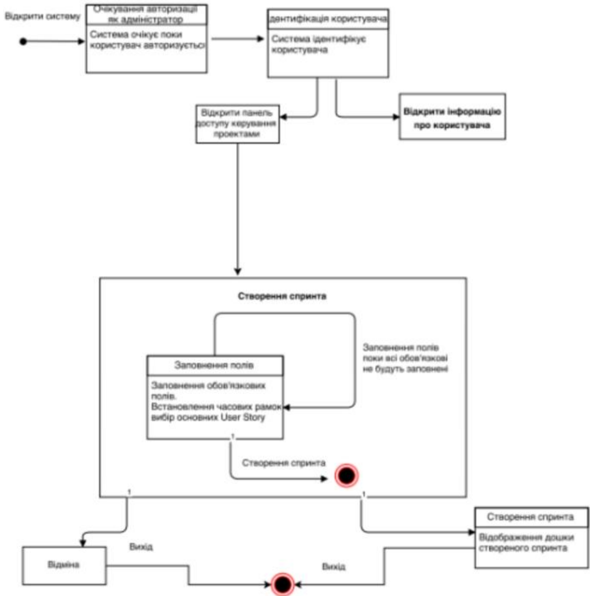
Рис. 2.4 – Діаграма станів для створення спринта
